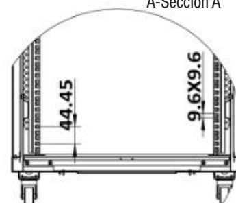
A-Sección A
