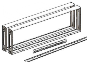
Caja 2: Marco del Armario Perfil de Montaje
