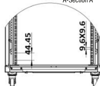
A-Section A
