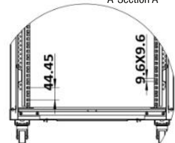
A-Section A
